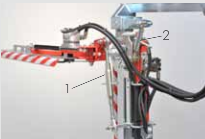
1 - Winkelverstellung des waagerechten Schneidbalkens 2 - Seitenneigung des kompletten Schneidwerks Hydraulische Verstellungen als Option
